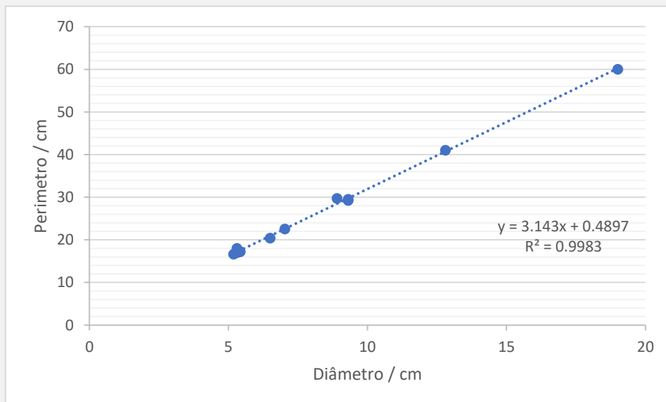
Gráfico 1. Determinação do valor de pi a partir do gráfico perímetro em função do diâmetro.
